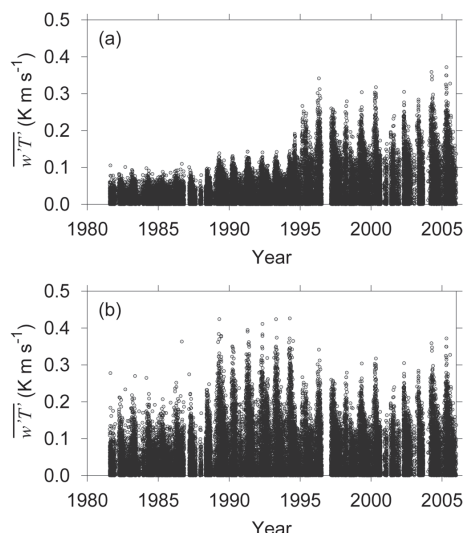
第5図 TERCで観測された顕熱フラックスの測定値(a)と1981年から1994年の間を補正したフラックス(b)。データは1時間平均値
