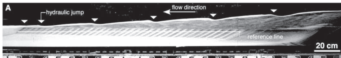
第3図 サイクリック・ステップの遡上により形成されたデルタ前置層の周期的粒径変化 (Muto et al. , 2012)
